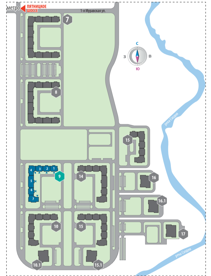
Генеральный план
