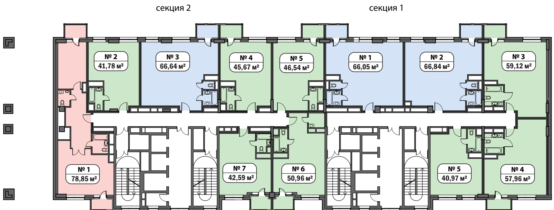
План 3-18 этажа
