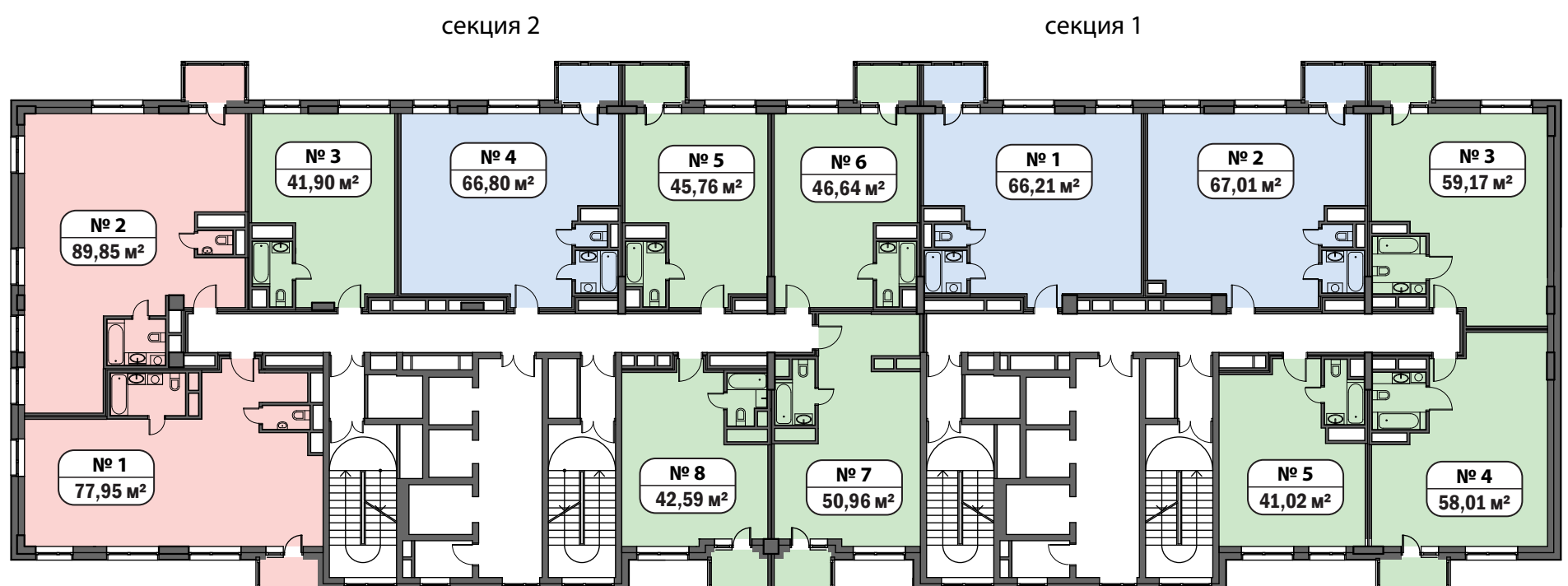
План 3-18 этажа
