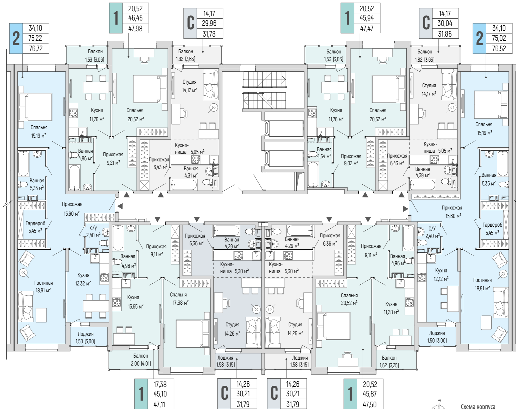
Схема корпуса
