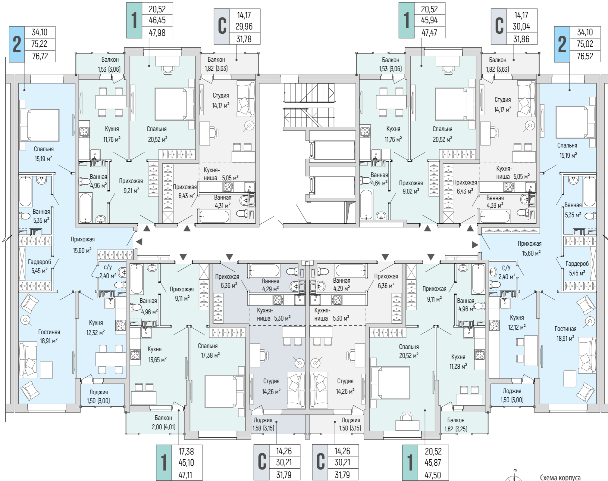
Схема корпуса
