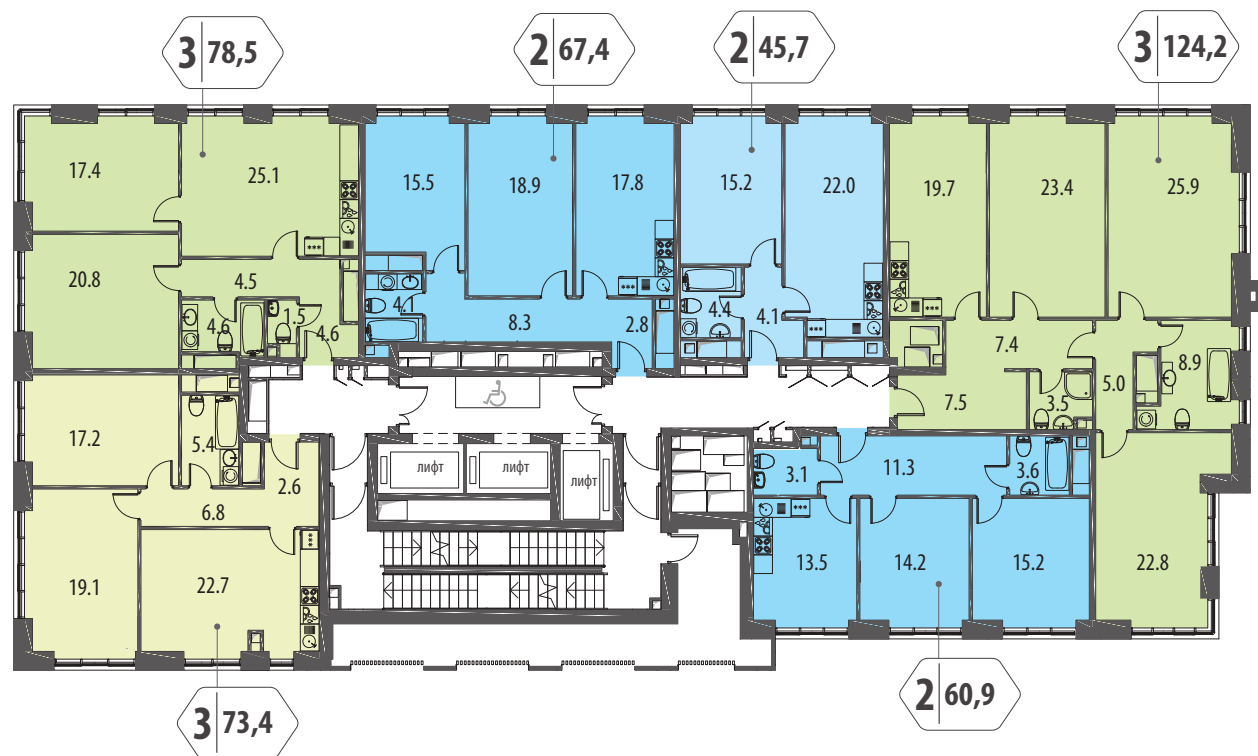
31-32 этаж
