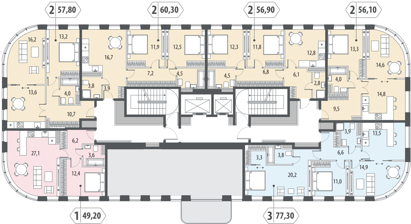
Планировочные решения 2 этаж.
