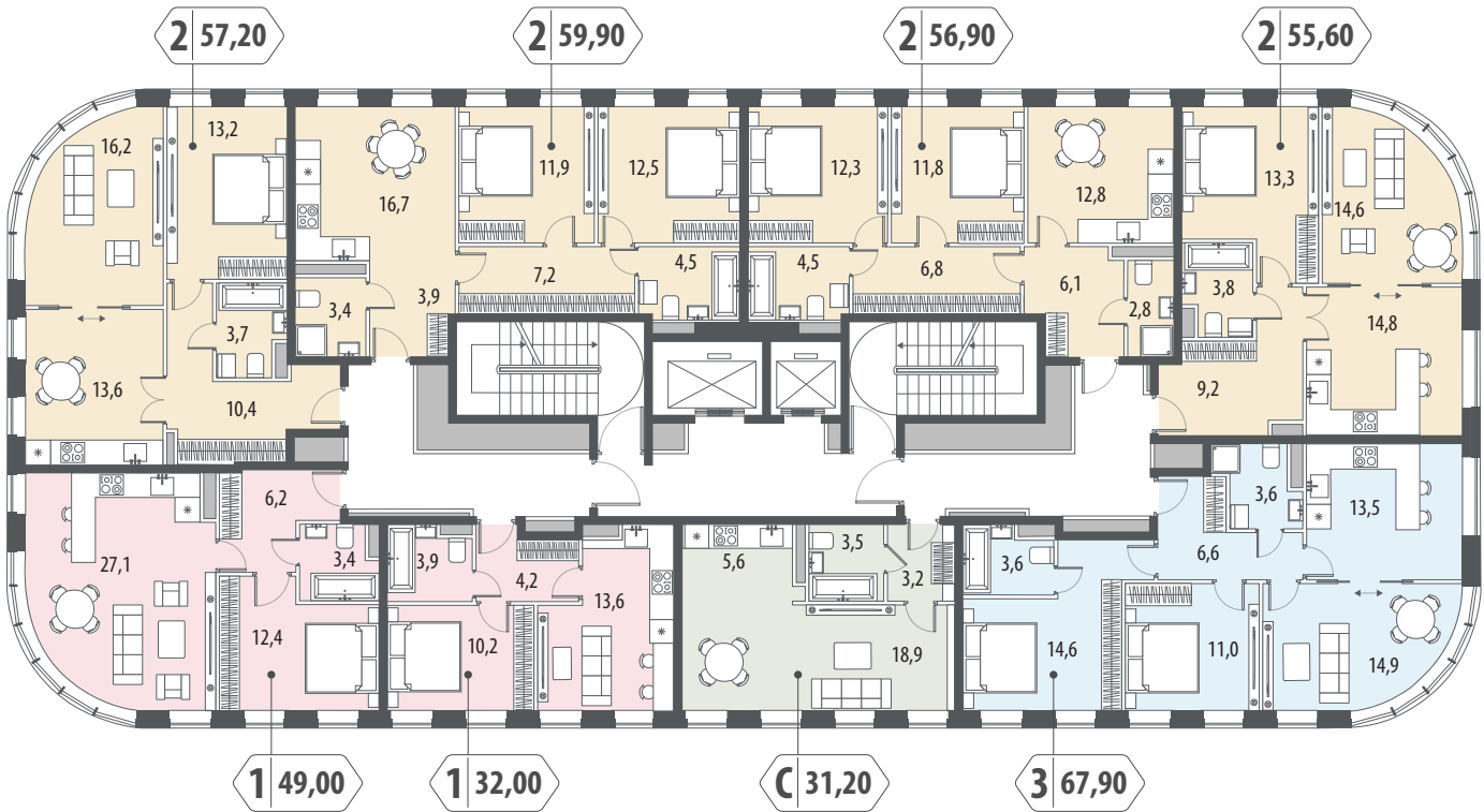
Планировочные решения 3-15 этаж.
